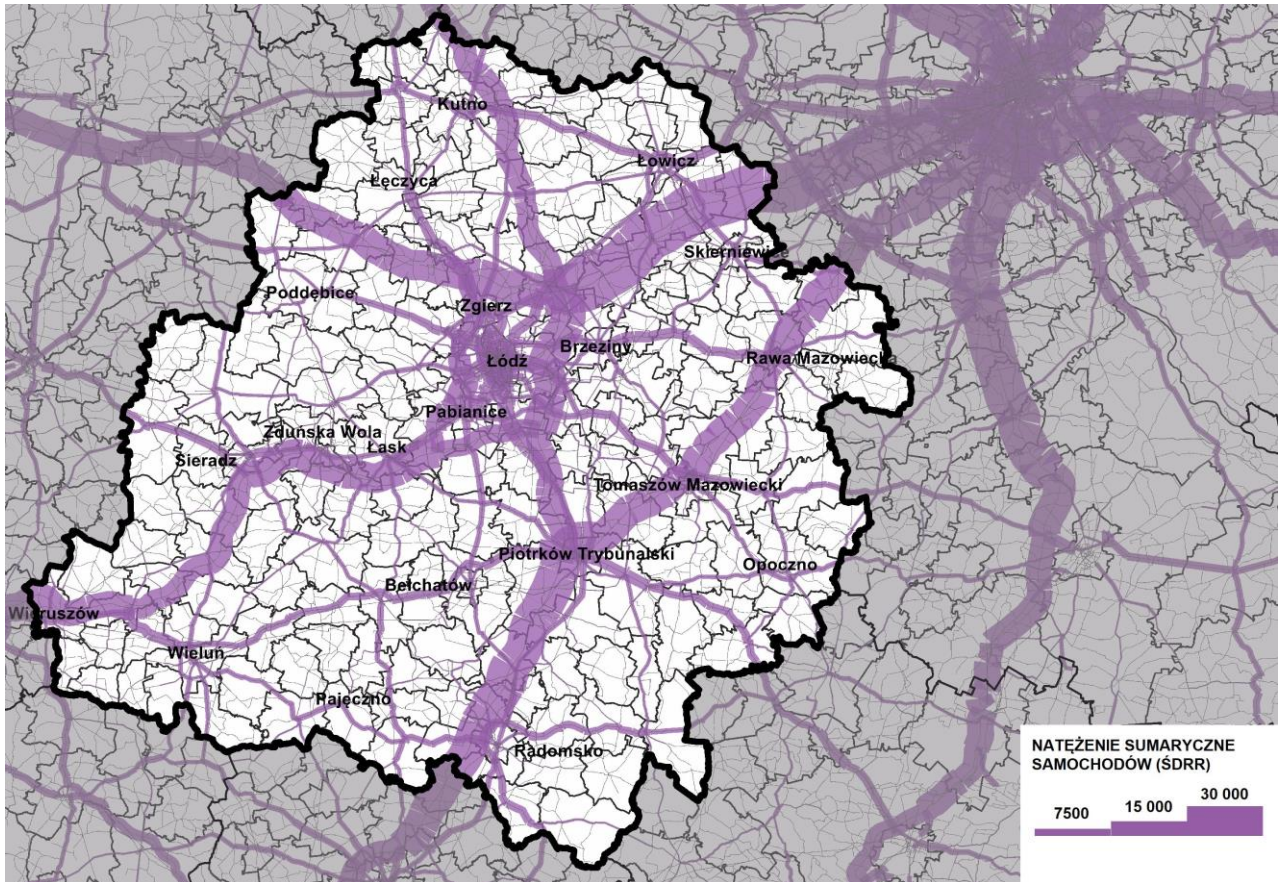
Rysunek 176 Scenariusz PTZ – Prognozowane natężenie ruchu pojazdów dla roku 2050 (Źródło: BPPWŁ we współpracy z IMS sp. z o.o. opracowanie własne na podstawie wyników analiz modelowania ruchu)
