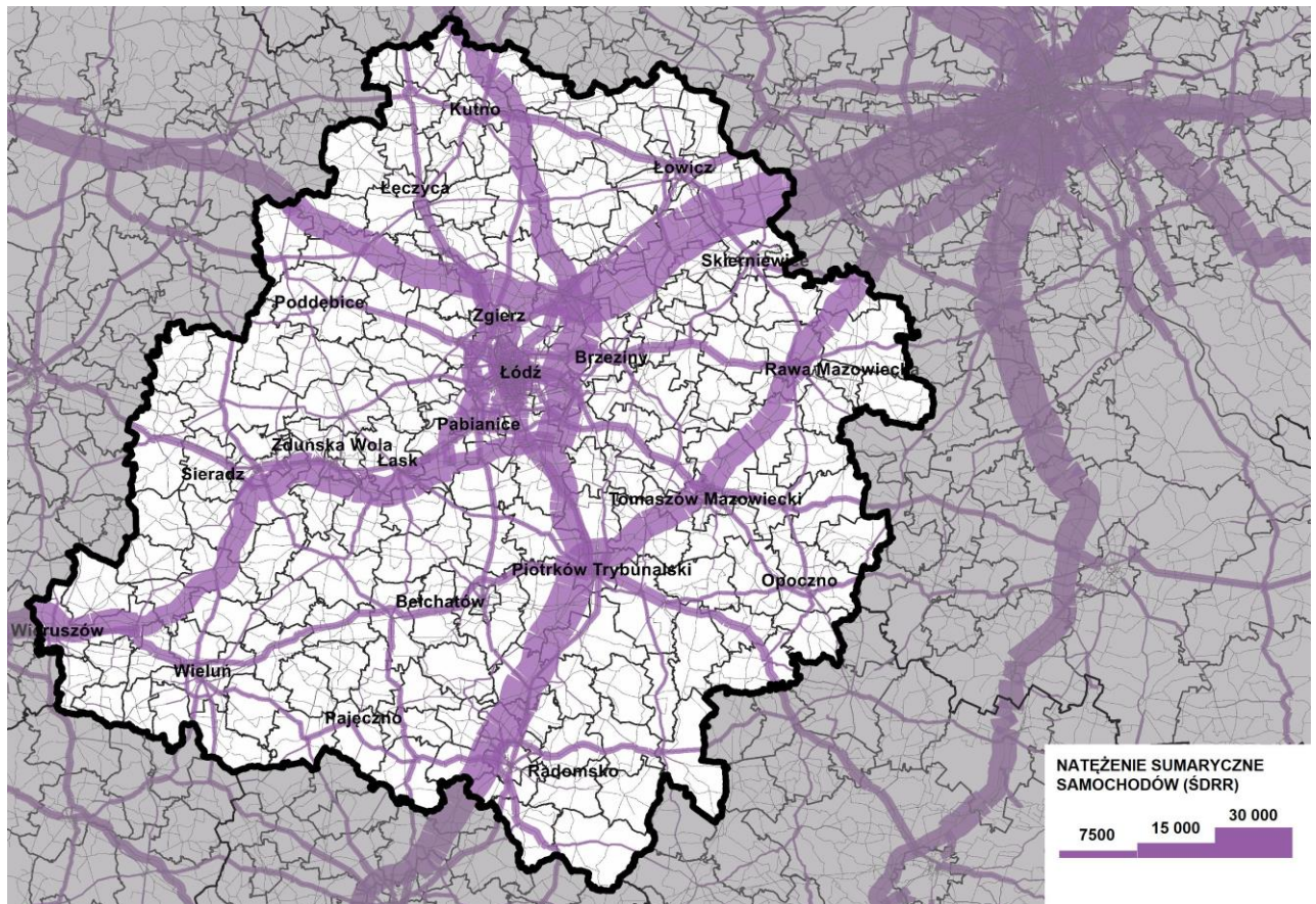
Rysunek 174 Scenariusz PTZ – Prognozowane natężenie ruchu pojazdów dla roku 2030 (Źródło: BPPWŁ we współpracy z IMS sp. z o.o. opracowanie własne na podstawie wyników analiz modelowania ruchu)
