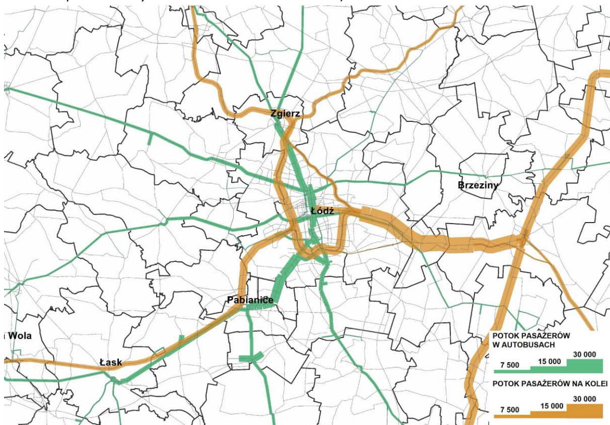
Rysunek 140 Rozkład potoków ruchu pasażerskiego na sieci transportowej województwa łódzkiego – obszar aglomeracji łódzkiej dla roku 2019 (Źródło: BPPWł we współpracy z IMS sp. z o.o. opracowanie własne na podstawie wyników analiz modelowania ruchu)
