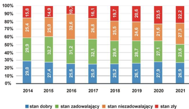
Rysunek 71 Stan nawierzchni dróg wojewódzkich w latach 2014–2021 (Źródło: BPPWŁ na podstawie Sprawozdań z przeprowadzonych przeglądów sieci DW administrowanych przez ZDW w Łodzi w latach 2014-2021)
