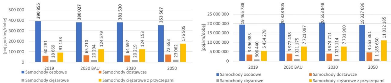
Rysunek 172 Scenariusz PTZ – zestawienie pracy przewozowej wyrażonej w pojazdogodzinach i pojazdokilometrach (Źródło: BPPWŁ we współpracy z IMS sp. z o.o. opracowanie własne na podstawie wyników analiz modelowania ruchu)
