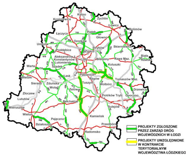
Rysunek 22 Przedsięwzięcia do realizacji zawarte w Planie Rozwoju Sieci Dróg Wojewódzkich (Źródło: BPPWŁ na podstawie PRSDW WŁ 2015-2023)
