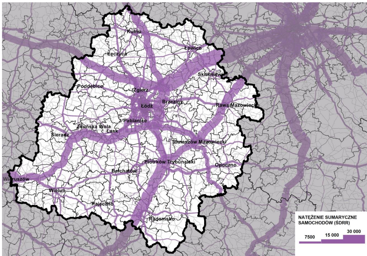
Rysunek 185 Scenariusz ZR – Prognozowane natężenie ruchu pojazdów dla roku 2030 (Źródło: BPPWŁ we współpracy z IMS sp. z o.o. opracowanie własne na podstawie wyników analiz modelowania ruchu)
