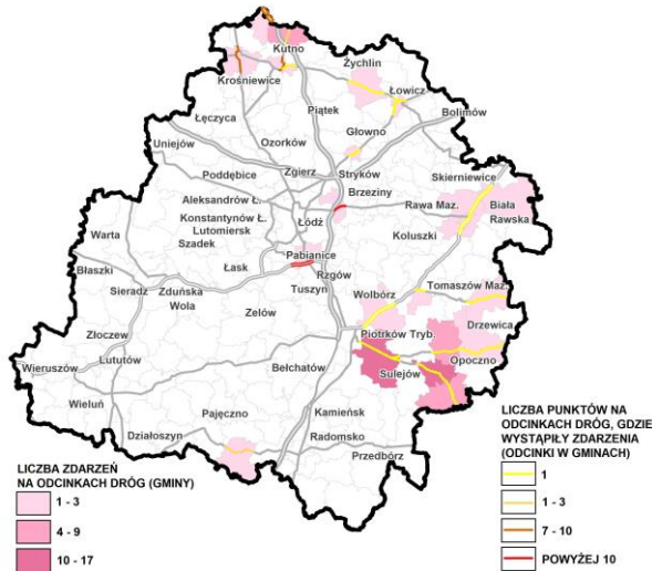
Rysunek 55 Odcinki dróg krajowych, na których w latach 2004-2015 występowały zdarzenia związane z silnymi opadami deszczu (Źródło: BPPWŁ na podstawie GDDKiA)
