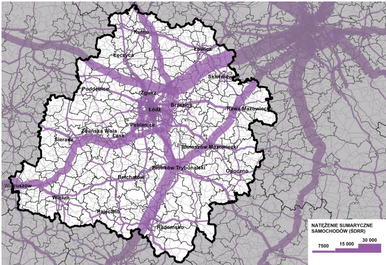
Rysunek 150 Scenariusz BAU – Prognozowane natężenie ruchu pojazdów dla roku 2030 (Źródło: BPPWŁ we współpracy z IMS sp. z o.o. opracowanie własne na podstawie wyników analiz modelowania ruchu)
