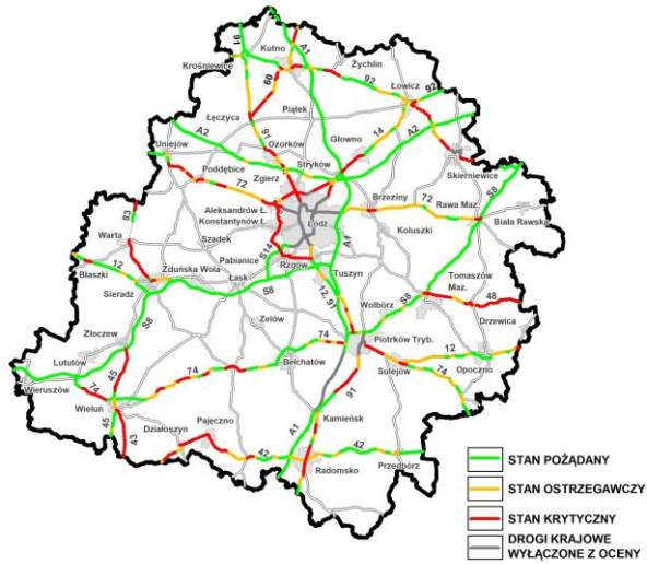
Rysunek 67 Stan nawierzchni dróg krajowych w 2021 r. (Źródło: BPPWŁ na podstawie Raportu o stanie nawierzchni sieci DK na koniec 2021)
