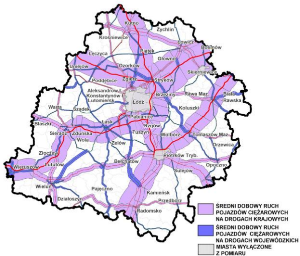
Rysunek 66 Natężenie ruchu pojazdów ciężarowych w 2020/2021 (Źródło: Opracowanie własne na podstawie GPR 2020/2021)
