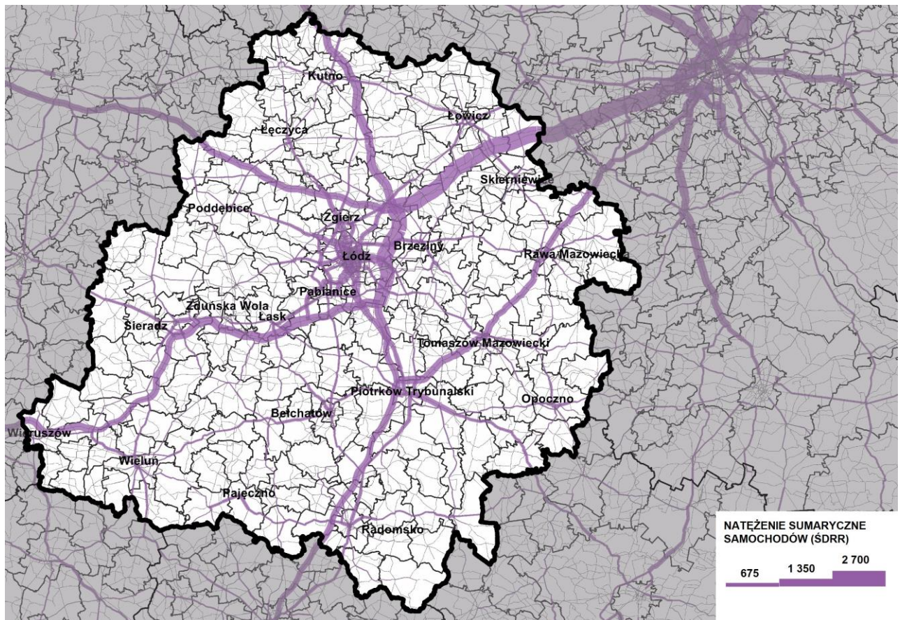
Rysunek 141 Rozkład ruchu drogowego na sieci dróg województwa łódzkiego w okresie szczytowym dla roku 2019 (Źródło: BPPWŁ we współpracy z IMS sp. z o.o. opracowanie własne na podstawie wyników analiz modelowania ruchu)
