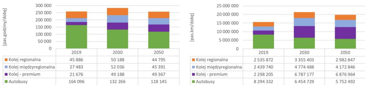
Rysunek 149. Scenariusz BAU – zestawienie pracy przewozowej wyrażonej w pasażerogodzinach i pasażerokilometrach (Źródło: BPPWŁ we współpracy z IMS sp. z o.o. opracowanie własne na podstawie wyników analiz modelowania ruchu)
