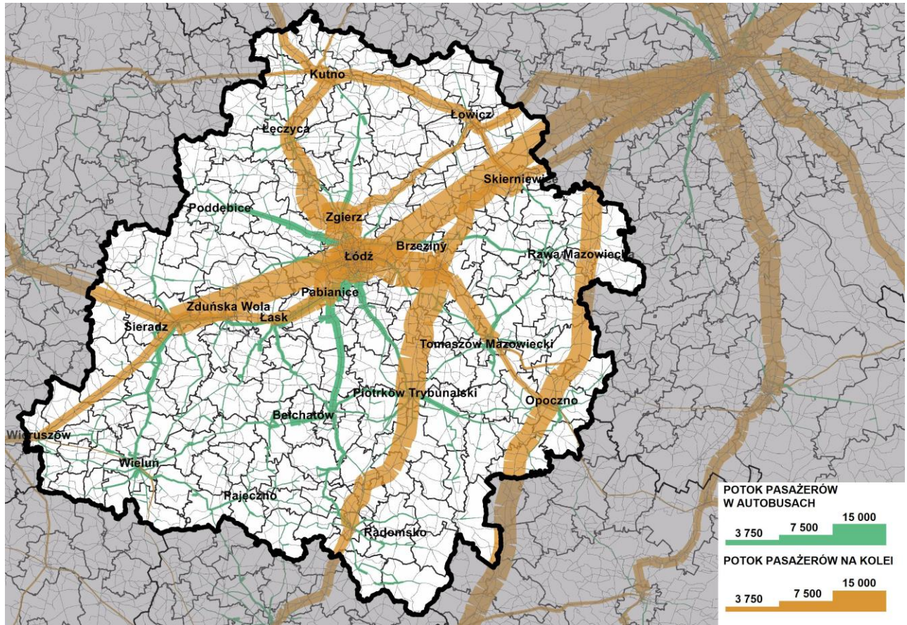
Rysunek 151 Scenariusz BAU – Prognozowane natężeniu ruchu pasażerów dla roku 2030 (Źródło: BPPWŁ we współpracy z IMS sp. z o.o. opracowanie własne na podstawie wyników analiz modelowania ruchu)
