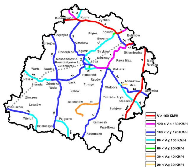
Rysunek 17 Prognoza na 2024 r. prędkości maksymalnych na liniach kolejowych zarządzanych przez PKP PLK SA (uwzględniająca efekty inwestycji kończonych w 2023 r.) w województwie łódzkim (Źródło: BPPWŁ na podstawie PFIK)
