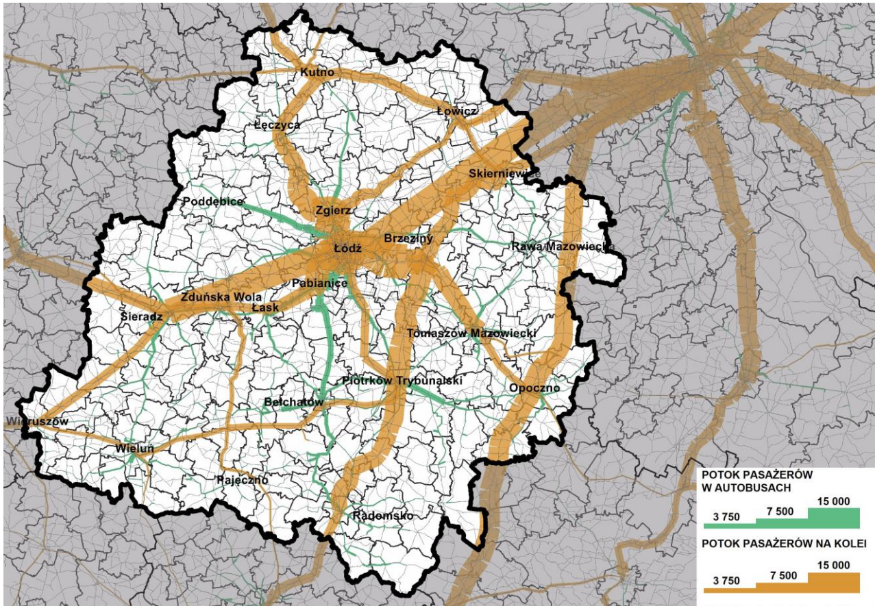
Rysunek 188 Scenariusz ZR – Prognozowane natężeniu ruchu pasażerów dla roku 2050 (Źródło: BPPWł we współpracy z IMS sp. z o.o. opracowanie własne na podstawie wyników analiz modelowania ruchu)
