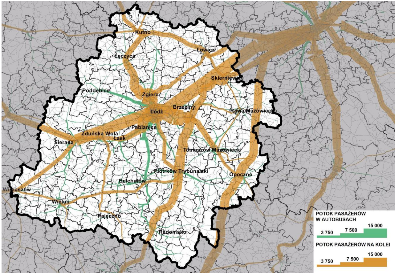
Rysunek 177 Scenariusz PTZ – Prognozowane natężeniu ruchu pasażerów dla roku 2050 (Źródło: BPPWŁ we współpracy z IMS sp. z o.o. opracowanie własne na podstawie wyników analiz modelowania ruchu)
