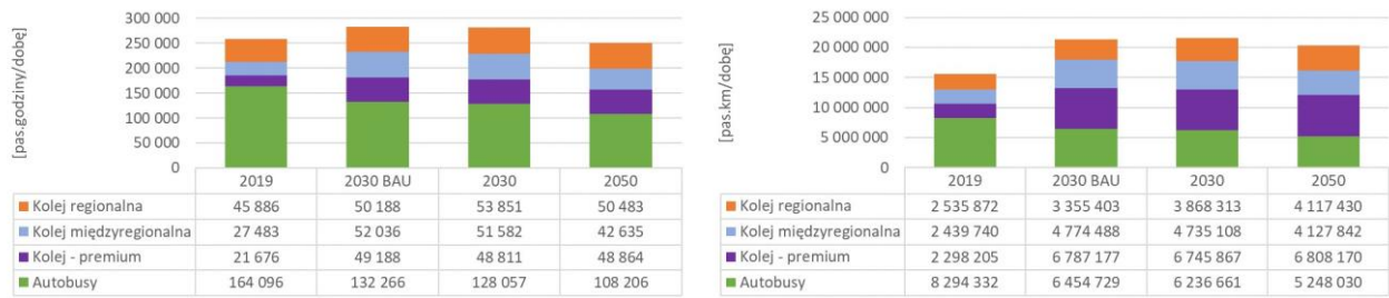
Rysunek 162 Scenariusz TI – zestawienie pracy przewozowej wyrażonej w pasażerogodzinach i pasażerokilometrach (Źródło: BPPWŁ we współpracy z IMS sp. z o.o. opracowanie własne na podstawie wyników analiz modelowania ruchu)
