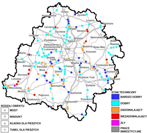
Rysunek 70 Ocena stanu technicznego obiektów inżynierskich w ciągu dróg wojewódzkich w 2021 r. (Źródło: BPPWŁ na podstawie Przeglądów rocznych ZDW w Łodzi)
