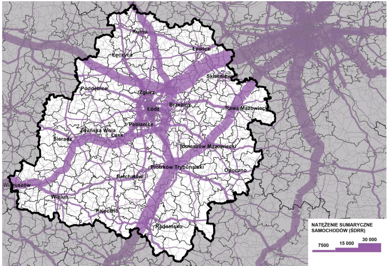
Rysunek 165 Scenariusz TI – Prognozowane natężenie ruchu pojazdów dla roku 2050 (Źródło: BPPWŁ we współpracy z IMS sp. z o.o. opracowanie własne na podstawie wyników analiz modelowania ruchu)
