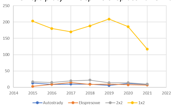
Rysunek 202 Liczba ofiar wypadków (zabitych) w zależności od typu i przekroju drogi w latach (Źródło: BPPWŁ we współpracy z IMS sp. z o.o. opracowanie własne na podstawie SEWiK)
