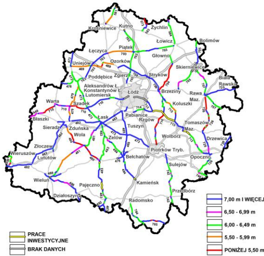
Rysunek 69 Szerokość jezdni dróg wojewódzkich w 2021 r. (Źródło: BPPWŁ na podstawie Przeglądów rocznych ZDW w Łodzi)
