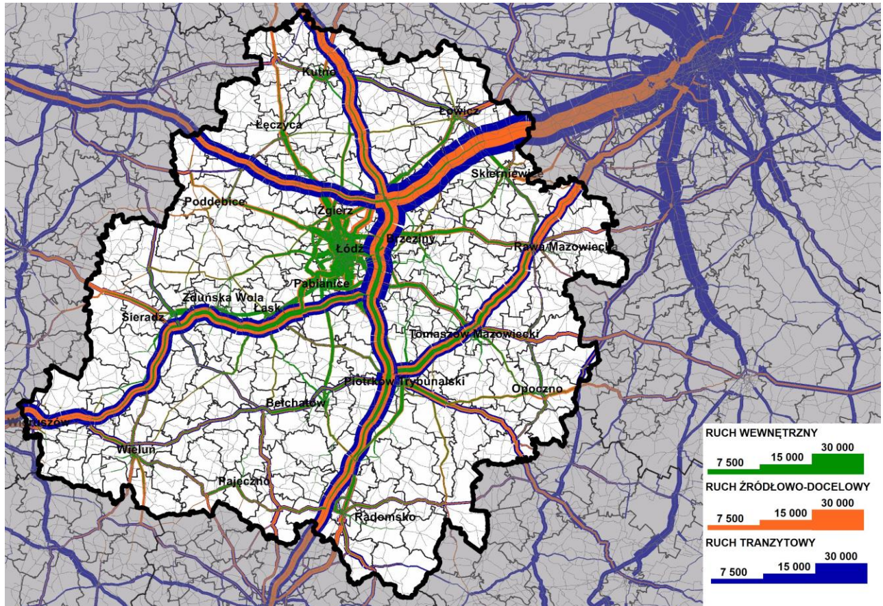
Rysunek 118 Rozkład ruchu tranzytowego, wewnętrznego i docelowego – transport indywidualny dla roku 2019 (Źródło: BPPWŁ we współpracy z IMS sp. z o.o. opracowanie własne na podstawie wyników analiz modelowania ruchu)
