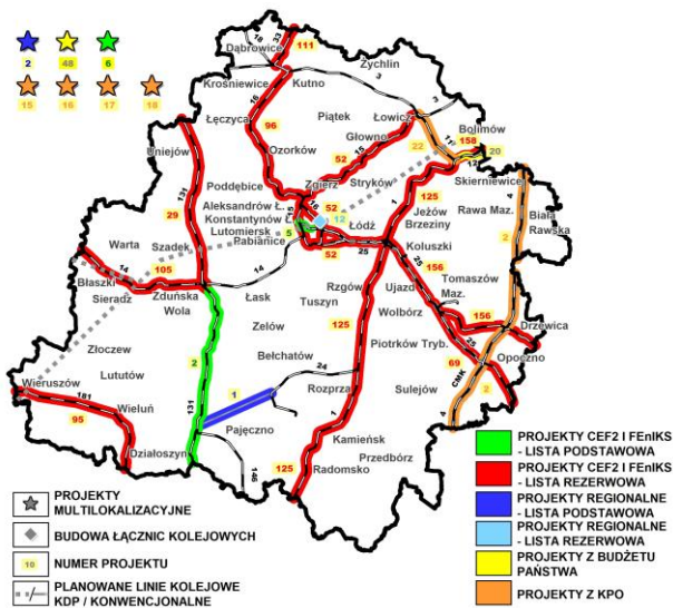
Rysunek 14 Zadania inwestycyjne w ramach Krajowego Programu Kolejowego po 2023 roku w województwie łódzkim (Źródło: BPPWŁ na podstawie KPK)
