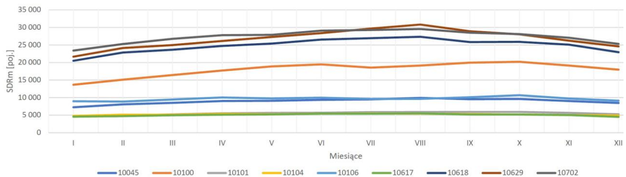
Rysunek 145 Sezonowe wahania ruchu dla roku 2019 (Źródło: BPPWŁ we współpracy z IMS sp. z o.o. opracowanie własne na podstawie danych z SCPR GDDKiA)
